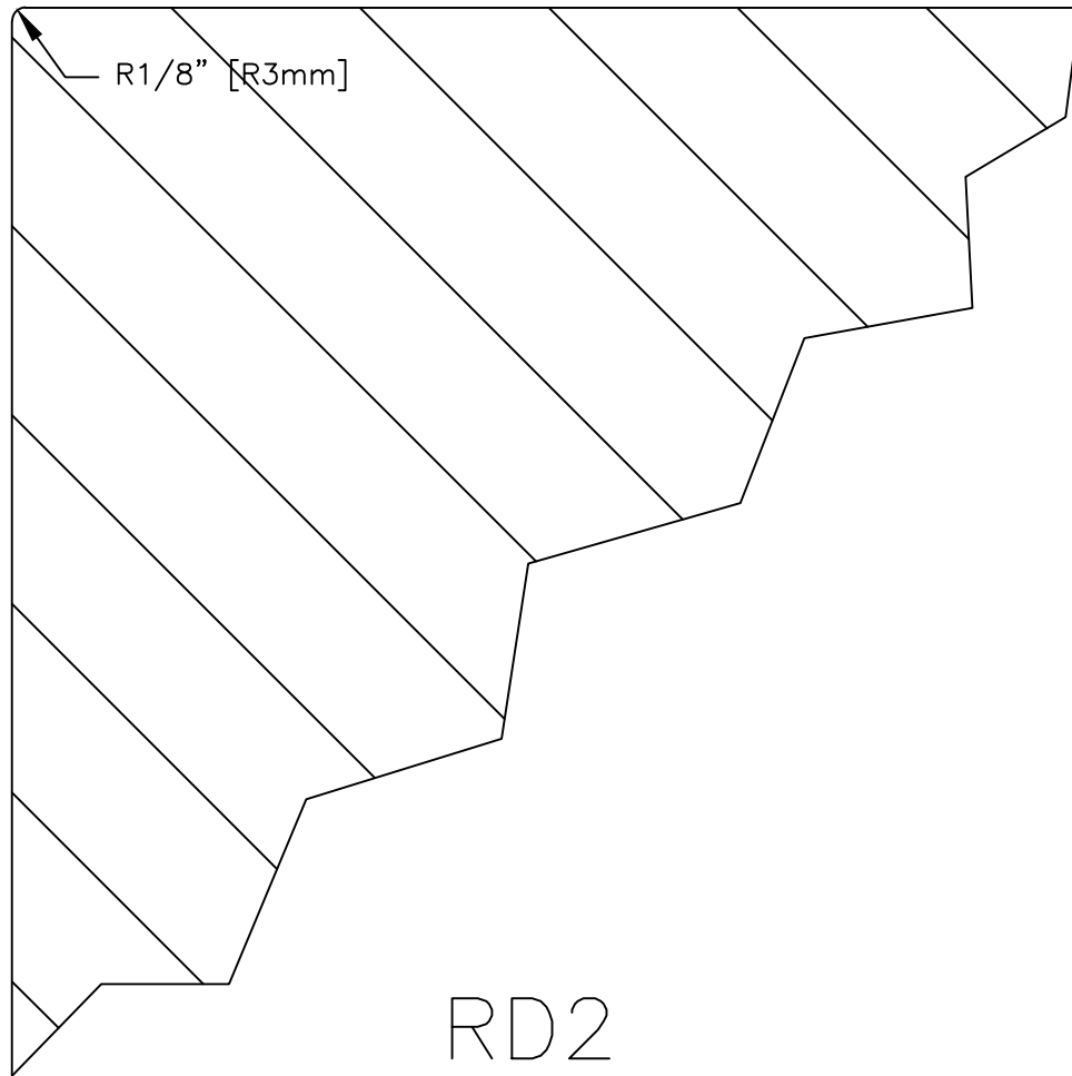
RD2 1/8" RADIUS EDGE SECTION
