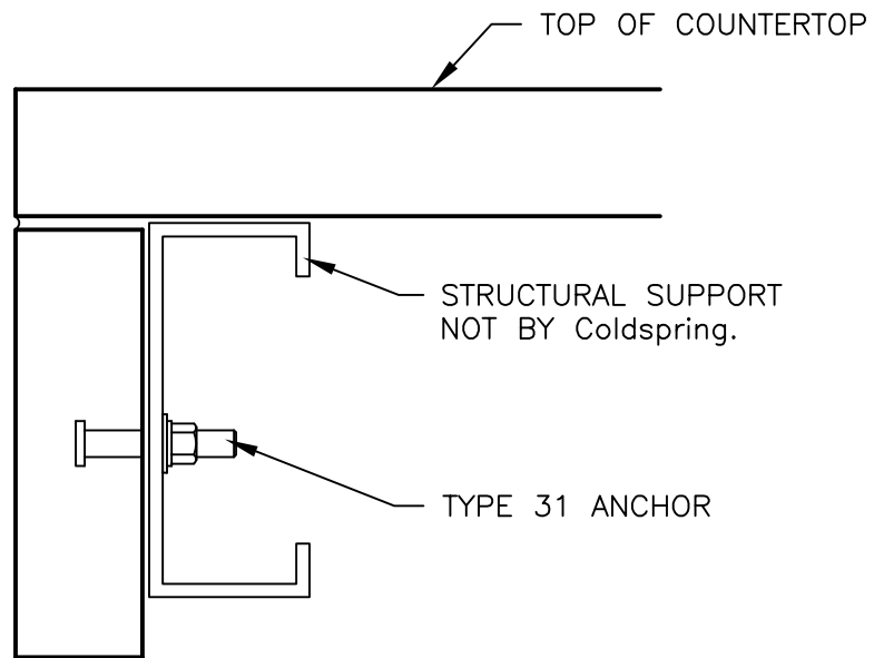
APRON SECTION
